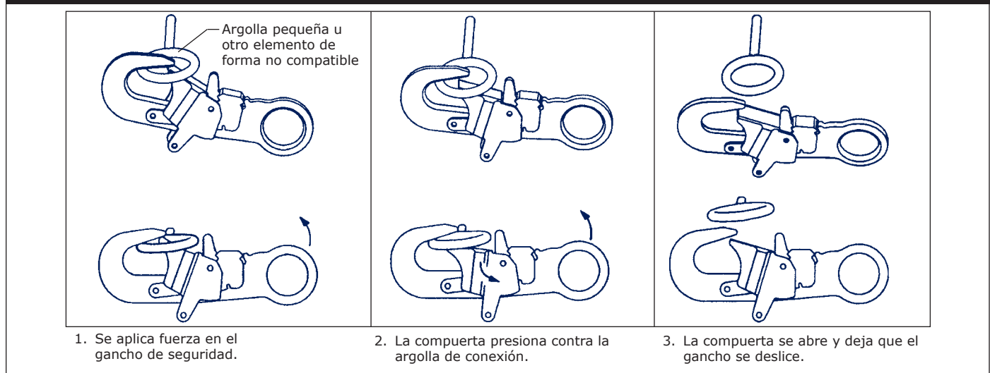
Figura 3: Desconexión accidental (deslizamiento)
