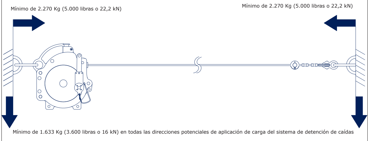
Figura 5: Resistencias del anclaje
