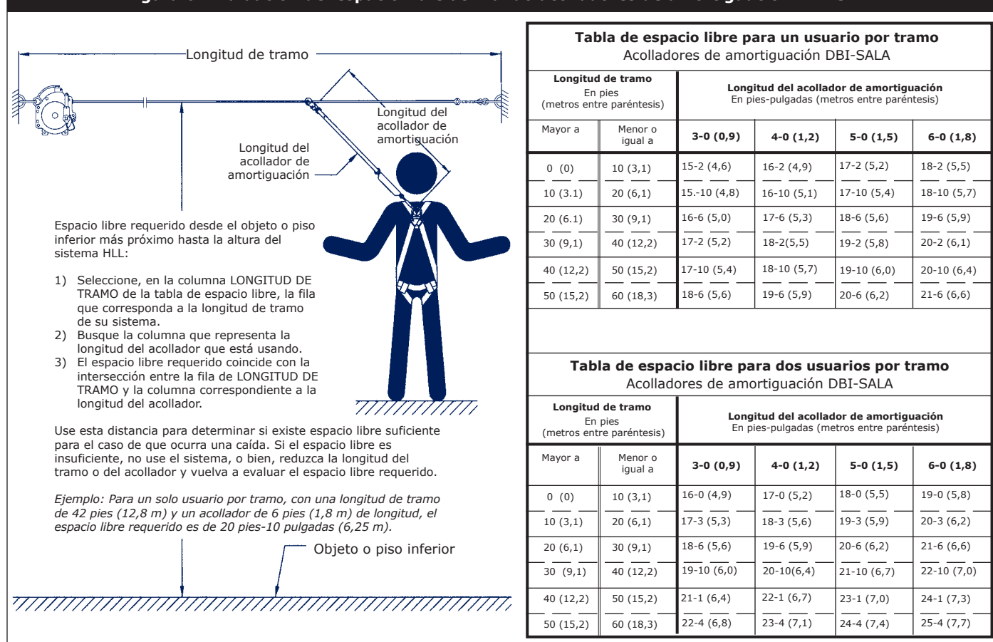
Figura 6: Evaluación del espacio libre utilizando acolladores de amortiguación DBI-SALA
