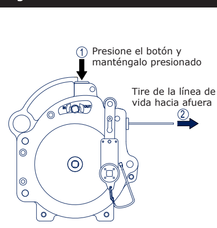
Figura 9: Tensión de la línea de vida
