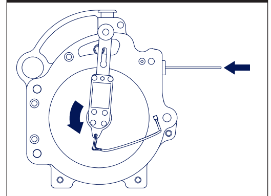
Figura 11: Retracción de la línea de vida
