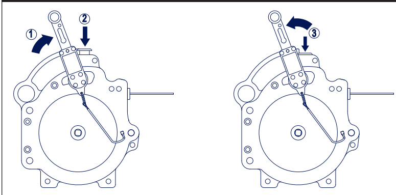
Figura 10: Aflojamiento de la línea de vida
