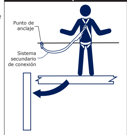
Figura 2: Riesgo de caída en movimiento pendular
