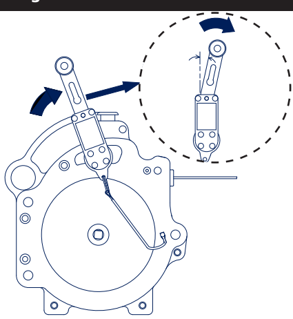
Figura 9: Tensión de la línea de vida
