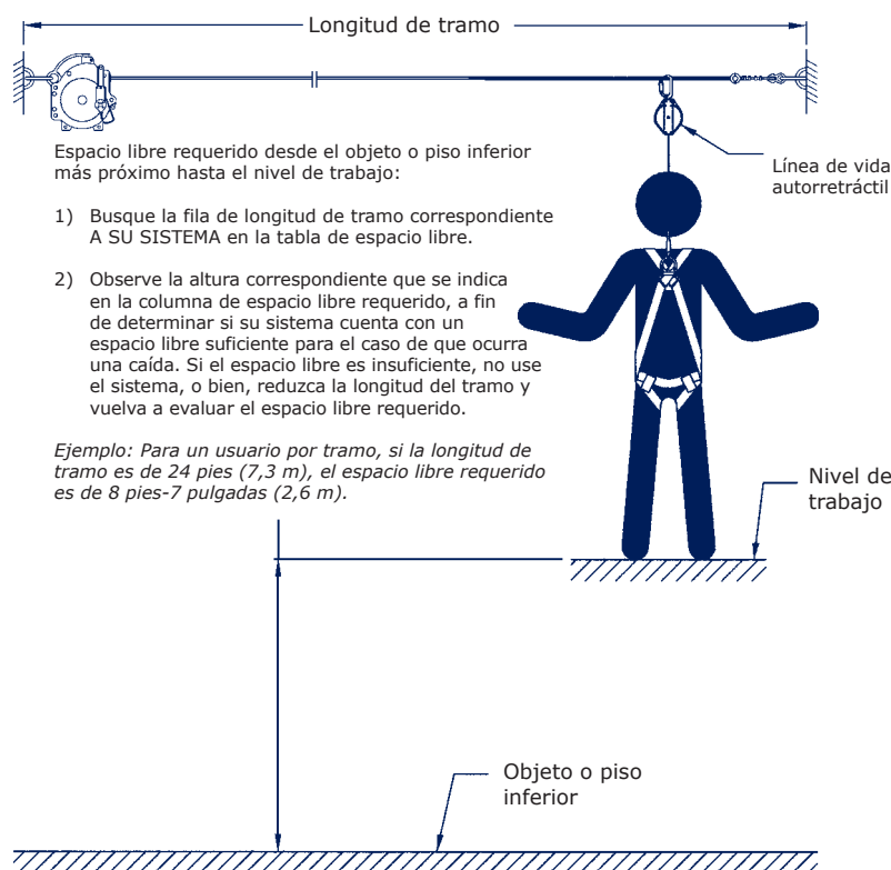
Figura 7: Evaluación del espacio libre utilizando líneas de vida autorretráctiles DBI-SALA
