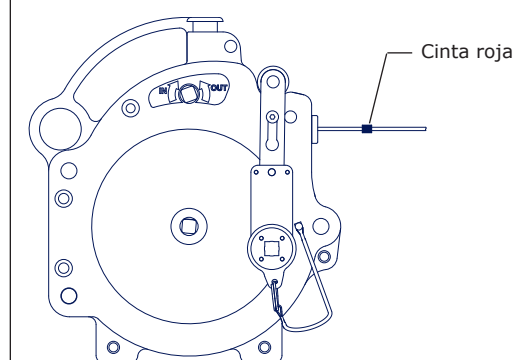
Figura 13: Indicador de extensión
