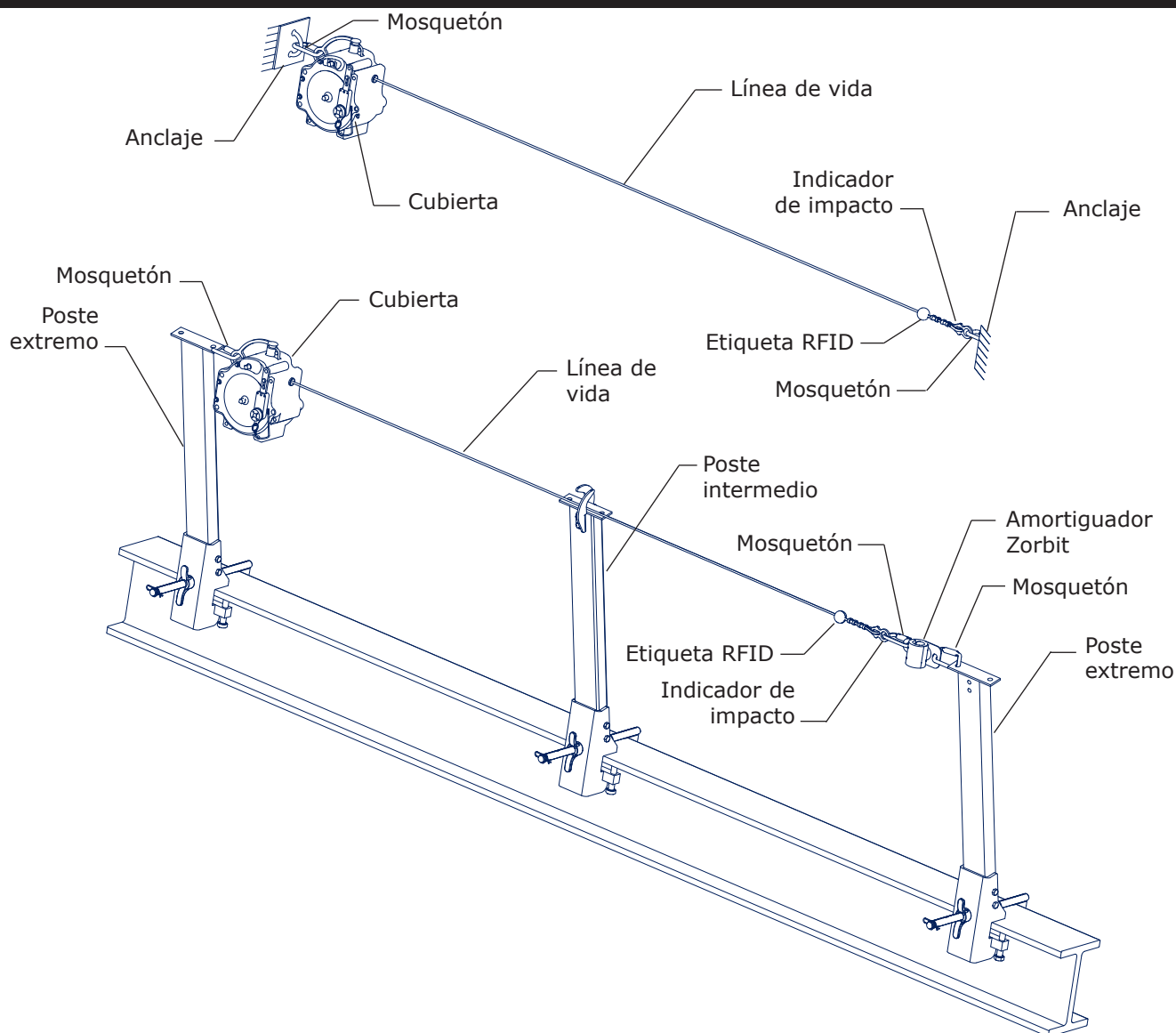
Figura 1: Configuración típica del sistema de línea de vida horizontal EZ-Line™
