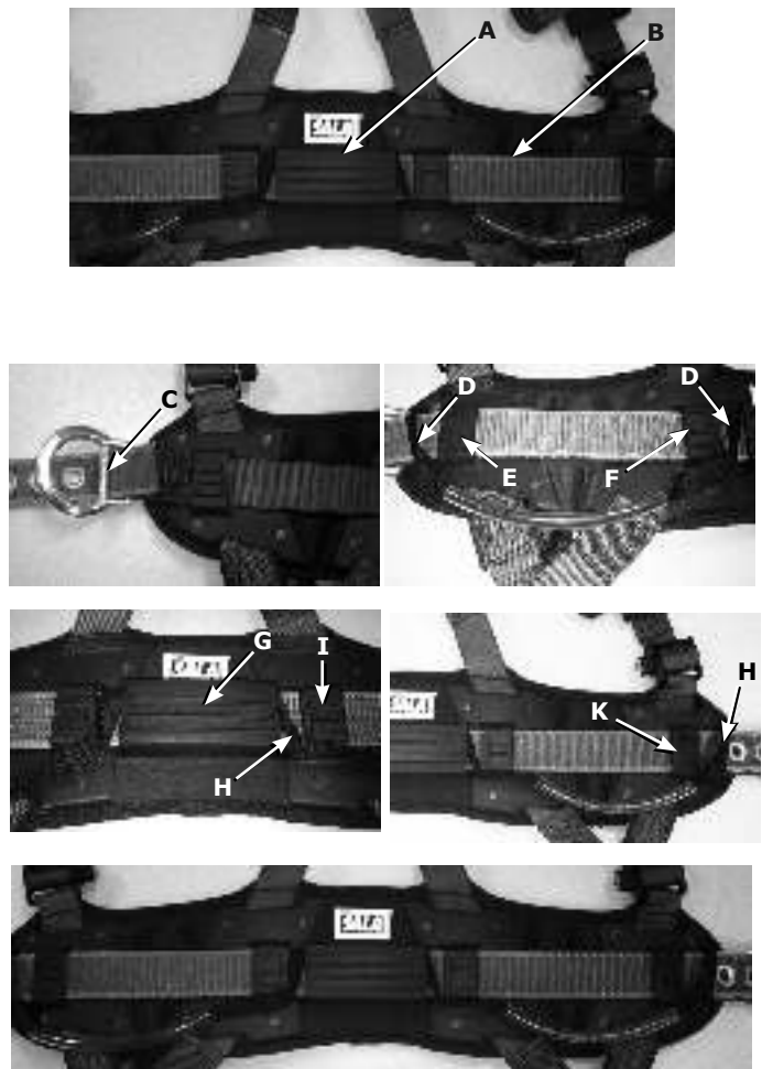
Figura 13 - Protector lumbar reemplazable
