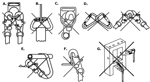
Figura 7 - Conexiones inapropiadas
