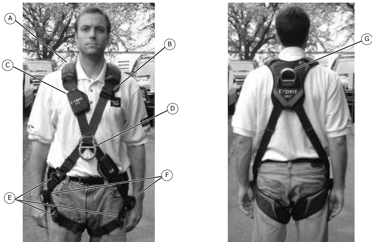
Figura 2: Arnés de cuerpo entero estilo cruzado ExoFit NEX™
